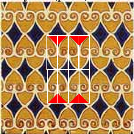
9 - sym 6 (pmm)
