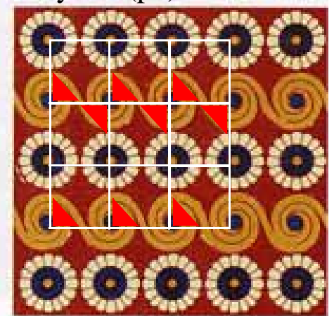
12 - sym 6 (pmm)
