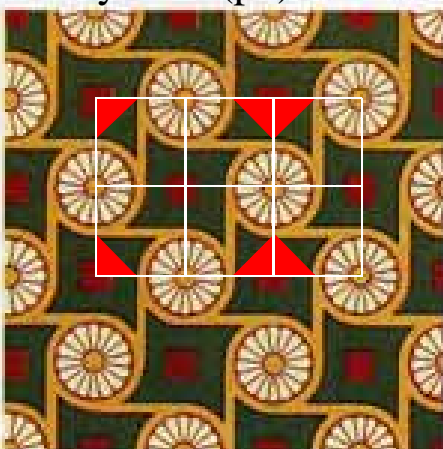
11 - sym 10 (p4)
