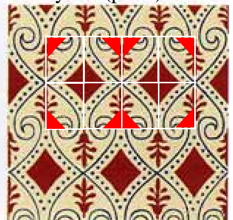
12 - sym 6 (pmm)
