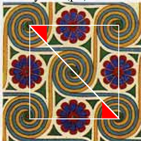
10 - sym 2 (p2)
