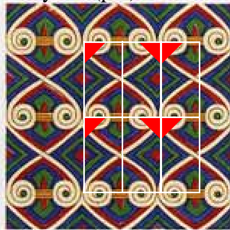
10 - sym 2 (p2)
