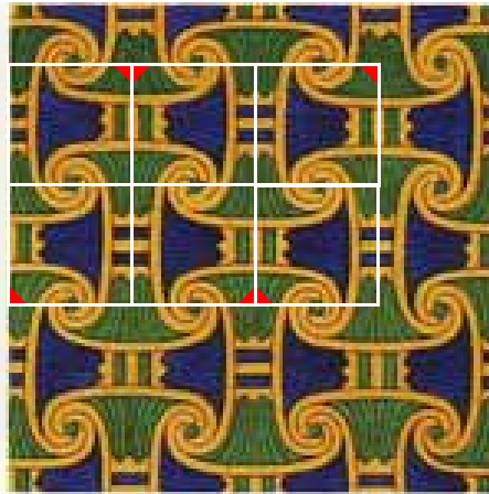
7 - sym 1 (p1)
